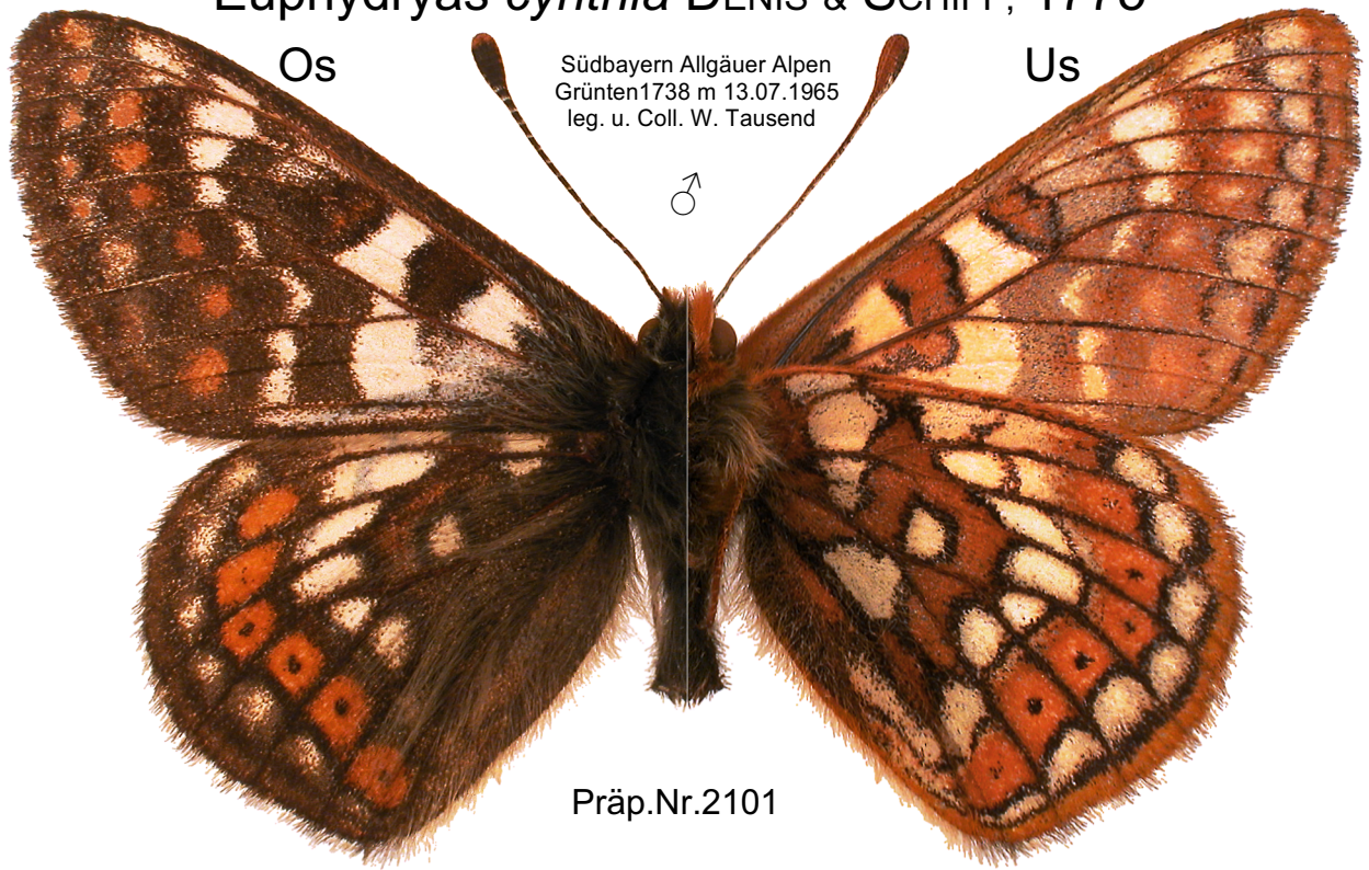
Genitalpräparat Nr. 2101
