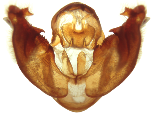
Kaudal-Ventralansicht Aed. sep. siehe Furca und Subscaphium
